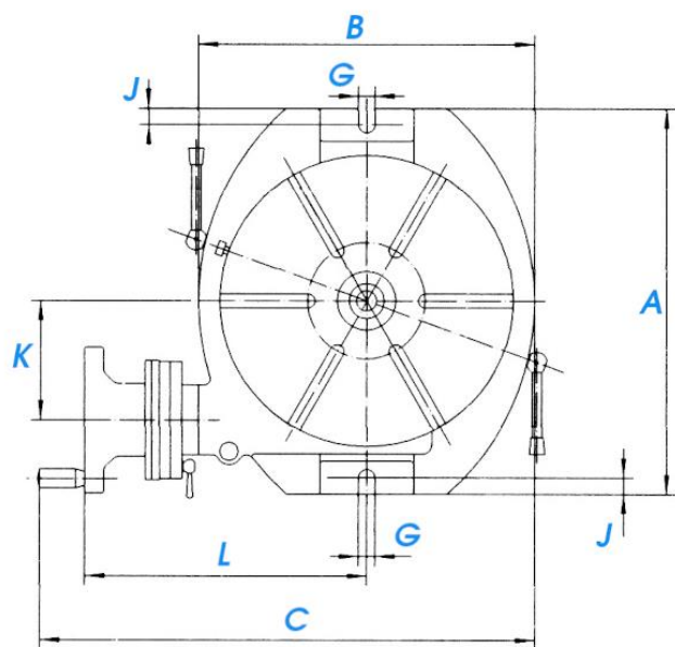
Столы поворотные ТИП 5030 TS..A
