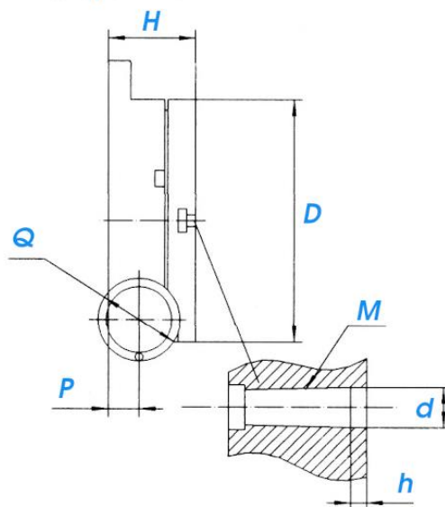
Столы поворотные ТИП 5030 TS..A
